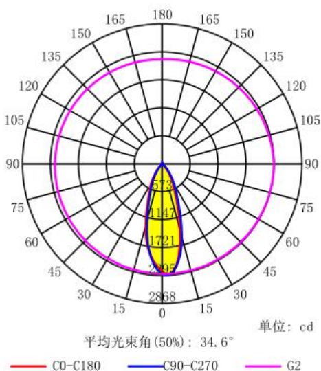
配光曲线
