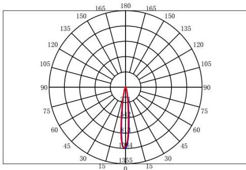
配光曲线
