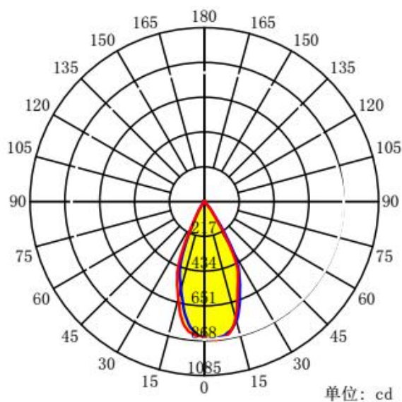
配光曲线
