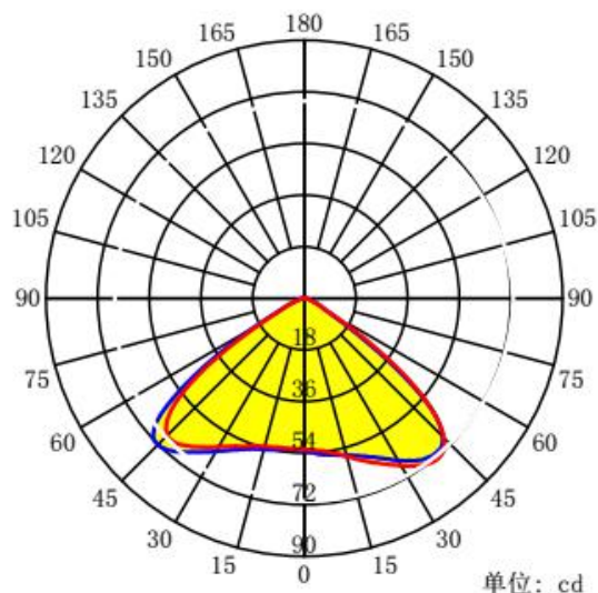
配光曲线
