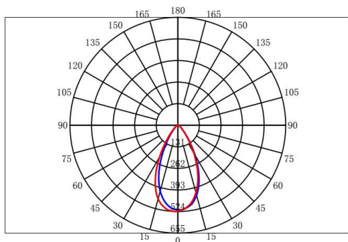
配光曲线
