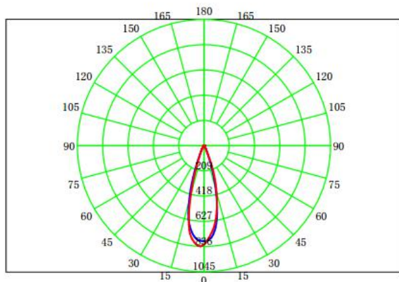
配光曲线
