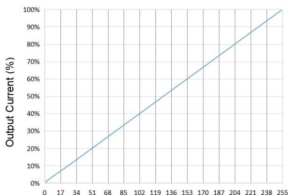
Linear dimming
