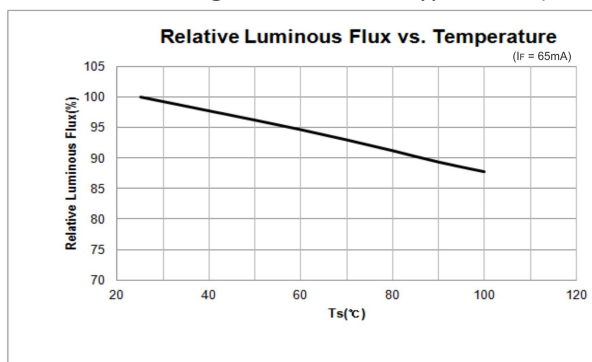
Температурные зависимости изменений светового потока и напряжения светодиодов Samsung Electronics типоразмера 5630 (серия 541MD)
