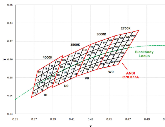
Хроматические координаты светодиодов Samsung Electronics типоразмера 5630 (серия 541MD)
