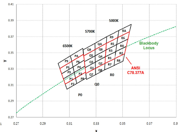
Хроматические координаты светодиодов Samsung Electronics типоразмера 5630 (серия 541MD)
