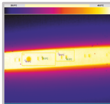
Термограмма, модуль NEO-L-16LS2835-280 ток 300 мА, Ta = 25°C, установившийся тепловой режим, без радиатора.
