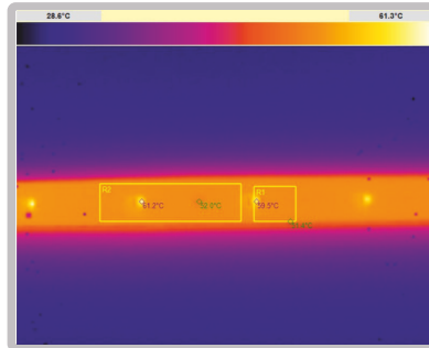
Термограмма, модуль NEO-L-18LS2835 ток 350 мА, Ta = 25°C, установившийся тепловой режим, без радиатора.
