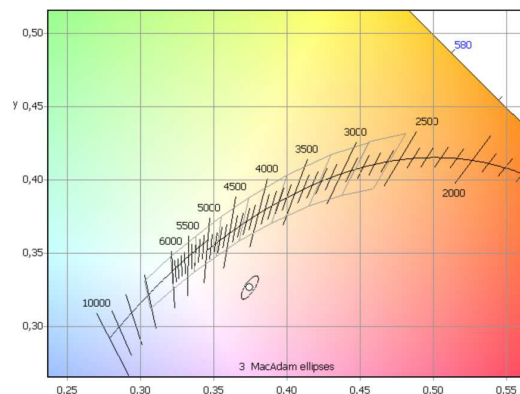
Спектральная плотность излучения и цветовые координаты светодиодов SEL-2835-YP435-3V350 SEL-2835-YP435-3V350 LEDs Spectral power distribution and Chromaticity coordinates, CIE
