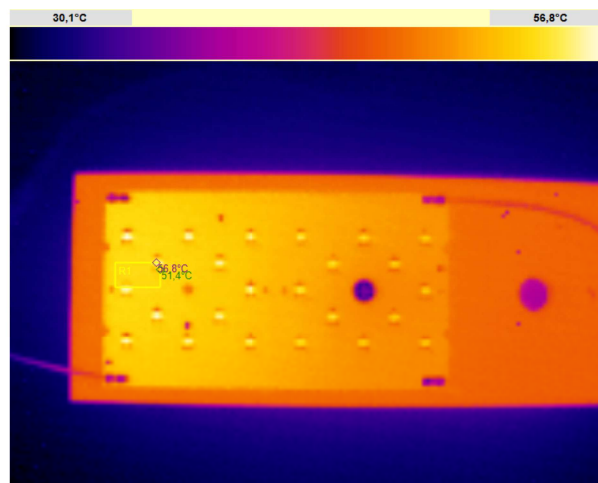
Термограмма NEO-L-24L3030, ток 350 мА T_a = 29^\circ\text{C} , установившийся тепловой режим, на радиаторе Step-72 (9 Вт). Thermogram NEO-L-24L3030, current - 350 mA T_a = 29^\circ\text{C} , steady thermal equilibrium, on a heatsink Step-72 (9 W).
