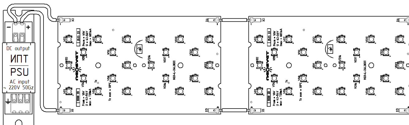
P.1 Параллельное включение / Parallel wiring of LED modules
