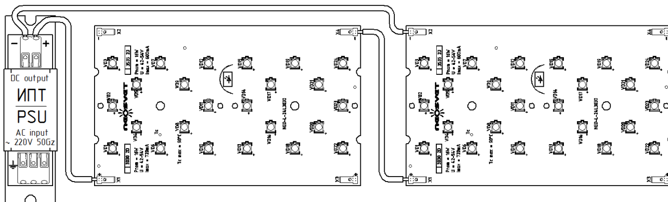
P.2 Последовательное включение / Serial wiring of LED modules
