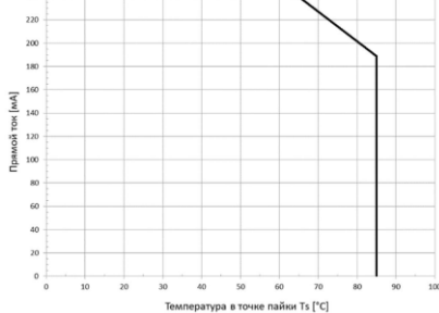
График области безопасной работы
