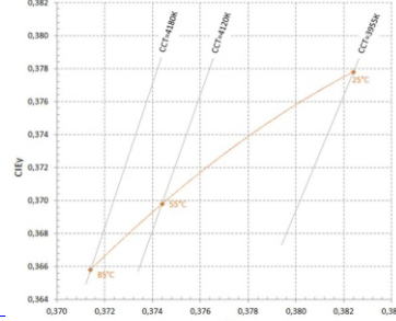
Типичная зависимость координат цветности от температуры T_s
