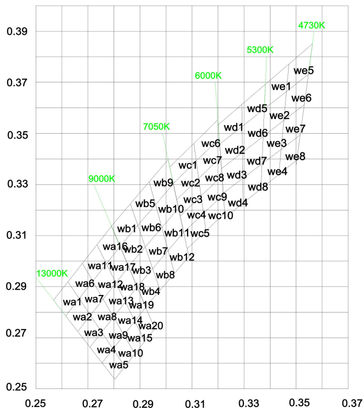
Хроматические координаты светодиодов SEL-2835-6V060. SEL-2835-6V060 LEDs type — 2835 Chromaticity Region & Coordinates
