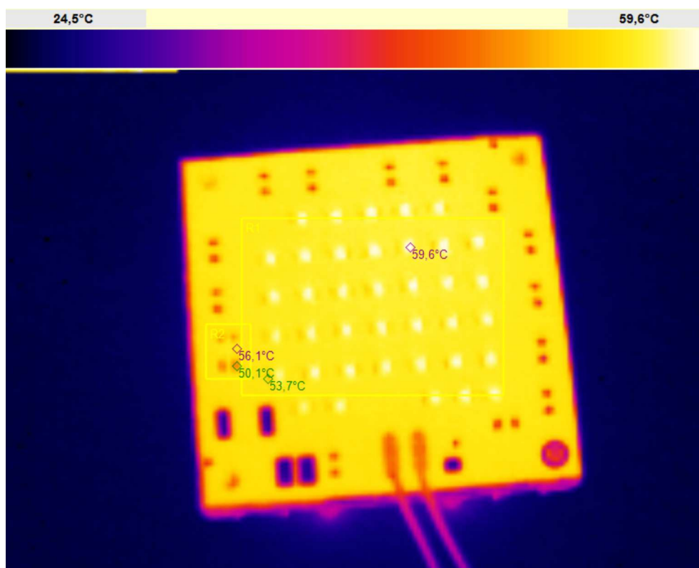
Термограмма NEO-Q-38S2835-AC. Питание от сети 230В 60Гц, T_a = 25^\circ\text{C} , установившийся тепловой режим, радиатор STEP-71. Thermogram NEO-Q-38S2835-AC. AC voltage 230 V 60 Hz., T_a = 25^\circ\text{C} , steady thermal equilibrium, heatsink STEP-71.
