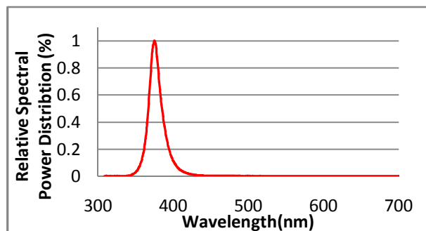
Fig.8- Spectrum Distribution 光谱分布特性曲线
