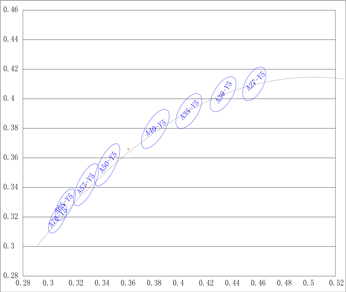
CIE Chromaticity Diagram 色区图
