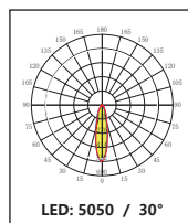
DK-5050-30-LENS-16H1
