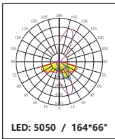
DK-5050-164X66-TPIII-M-4H1
