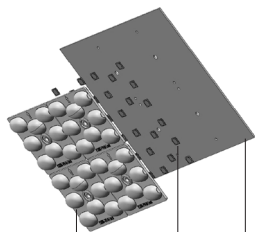
透镜 Lens 光源 LED CHIP 铝基板 PCB
