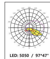
DK-5050-97*47-TPIV-4H1
