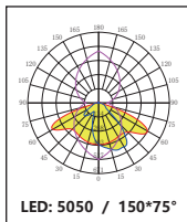
DK-173-160*80-TPII-M-V-12H1-5050-B
