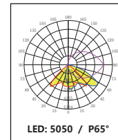
DK-5050-P65-REF-4H1-TSL-D1
