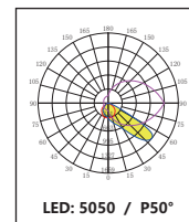
DK-5050-P50-LENS-6H1-NN1
